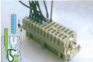
Step 2:将线端插入圆形接口。
