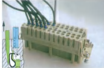
Step 3:取出螺丝起子，弹片收回原位，从而夹紧 插入的线端。
