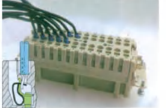
Step 4:连接完成，请拉动线端以确认线端确 实被弹片夹紧。
