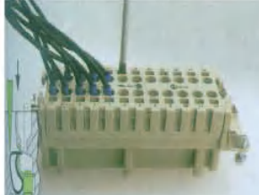
Step 1:螺钉起子插入正方形插孔中，弹片被 推向一侧，从而打开接线口。
