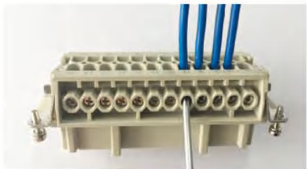
Step 4:连接完成，请拉动线端以确认线端确 实被弹片夹紧。
