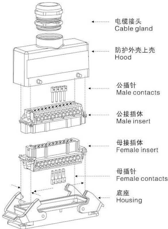
接插件安装示意图 Assembly details
