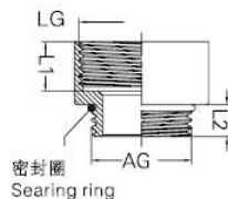
圆形金属扩径环 Round metal enlargement
